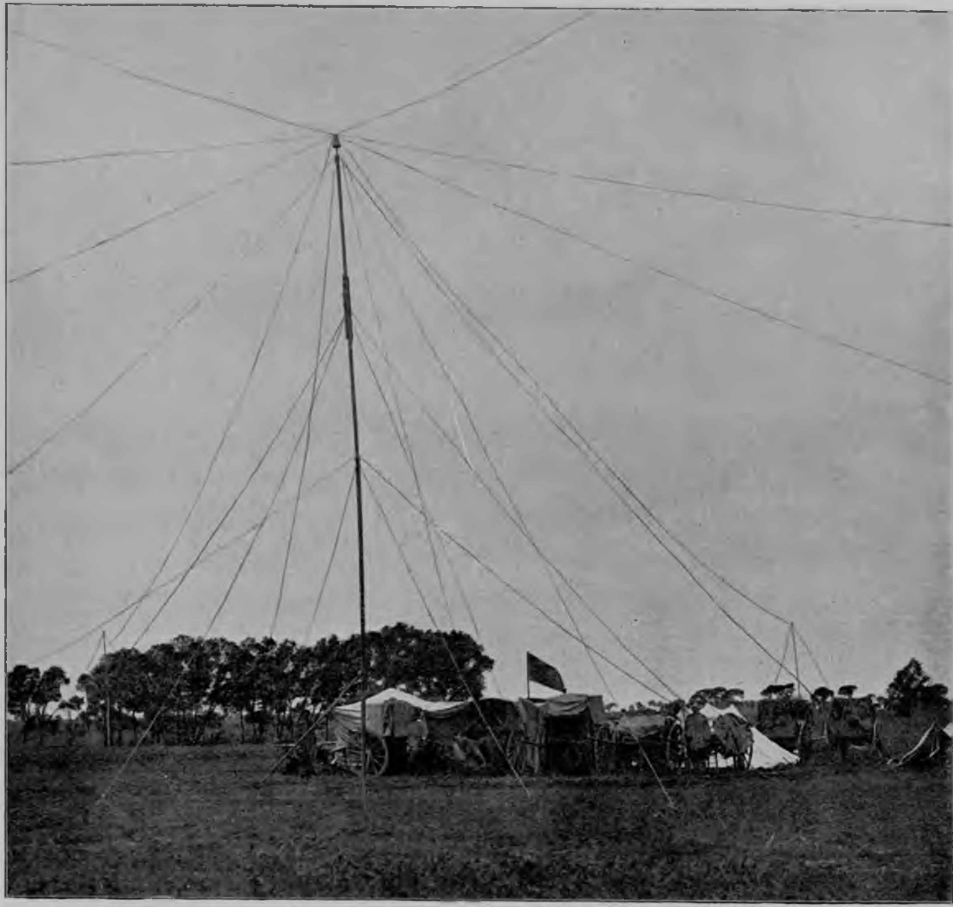
Станція безпроводного телеграфа въ д. Людяпудзы.
